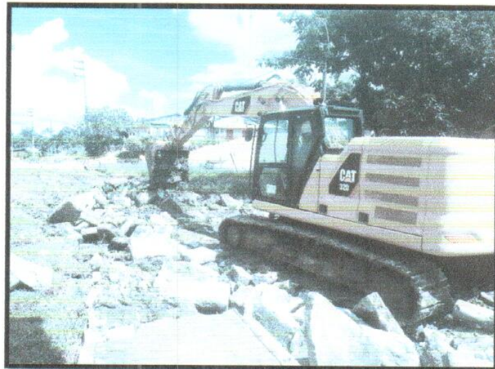
DEMOLICIÓN DE VEREDA EXISTENTE
