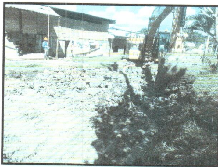
CONSTRUCTORA E INMOBILIARIA AMAZONICA E.I.R.L. CORTE A NIVEL DE SUBRASANTE EN LA PROGRESIVA 0+460
