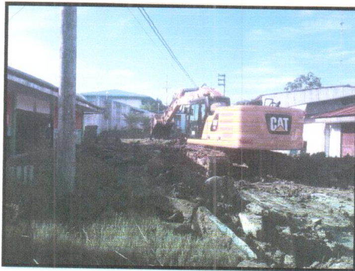
CORTE A NIVEL DE RASANTE EN LA PROGRESIVA 0+260
