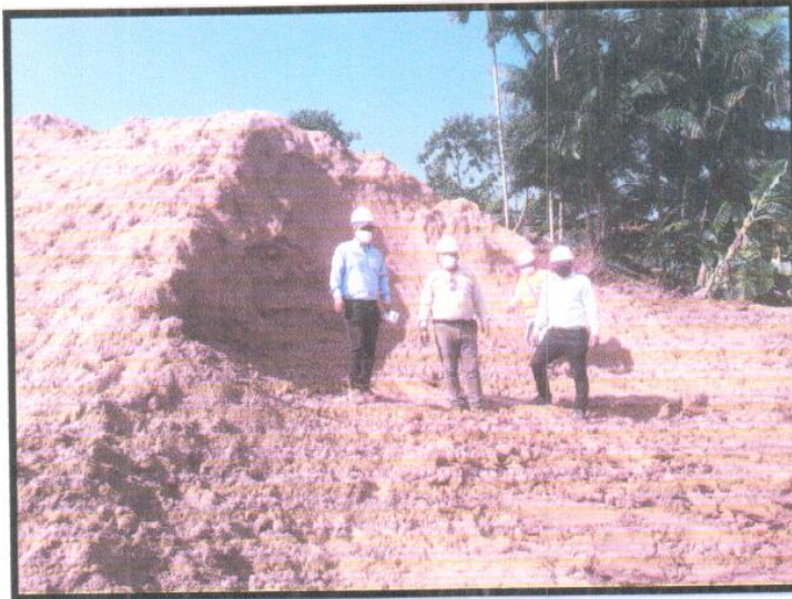
VERIFICACIÓN DE MATERIAL (CANTERA) A UTILIZARSE EN OBRA
